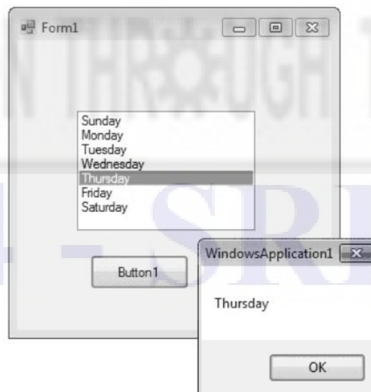
Fig. 3.11 List Box
