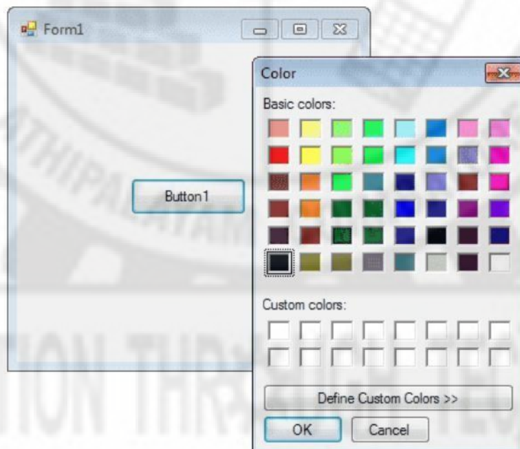
Fig. 3.43 Color Dialog
