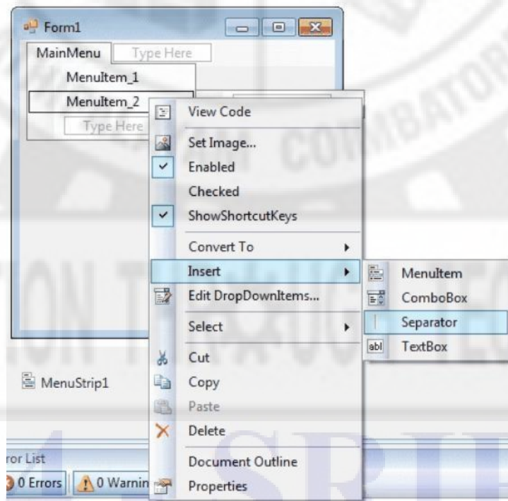
Fig. 3.41 Adding separator
