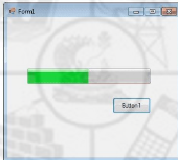
Fig. 3.17 Progress Bar
