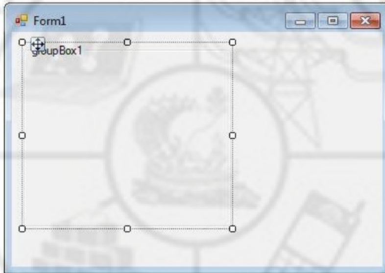
Fig. 3.15 GroupBox
