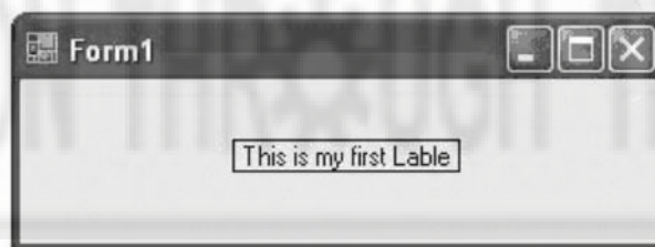
Fig. 3.7 Label
