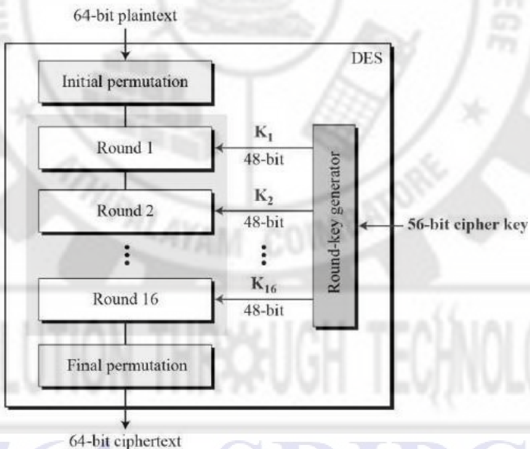
Fig 4.1 : DES Structure
