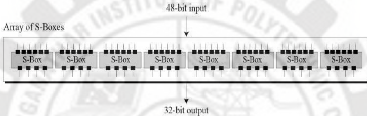
Fig 4.5 : Substitution Boxes
