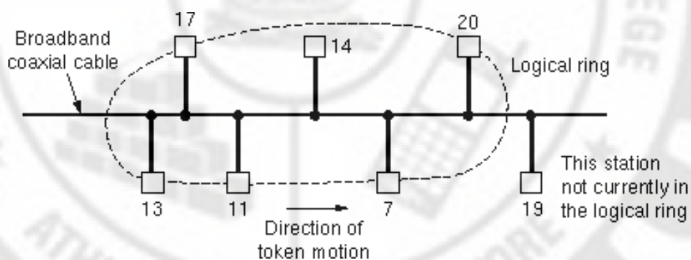
Fig 2.4 : Token Bus (802.4)
